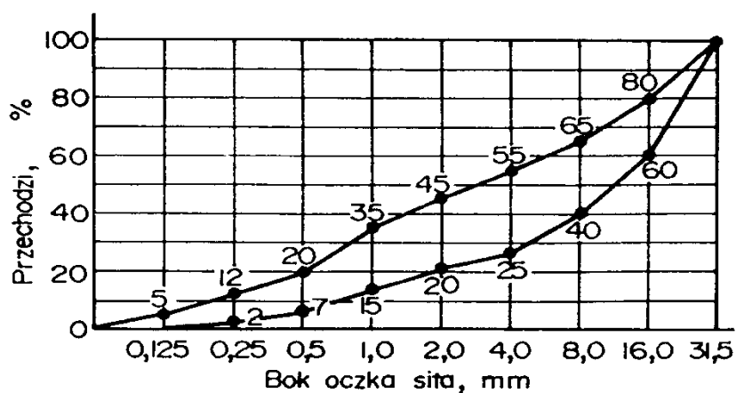
Rys. 1. Krzywe graniczne uziarnienia kruszywa do chudego betonu kruszywa od 0 do 31,5 mm
