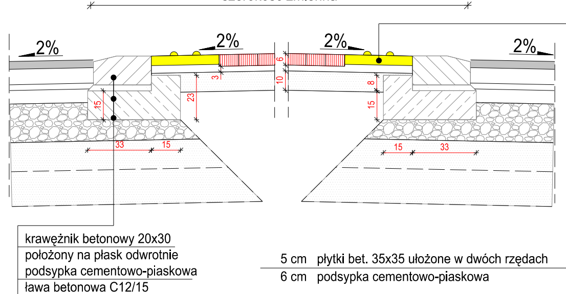
Szczegół wykonania wyspy dzielącej z przejściem dla pieszych
