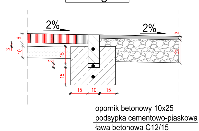
Szczegół 5
