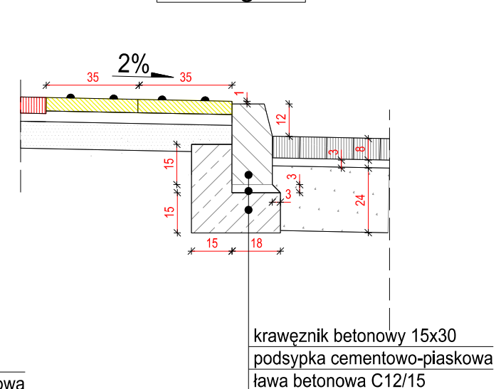
Szczegół 3
