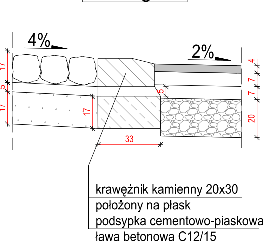
Szczegół 8
