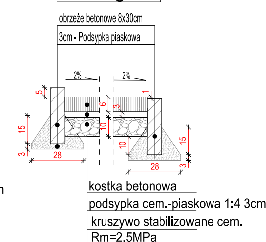
Szczegół 7
