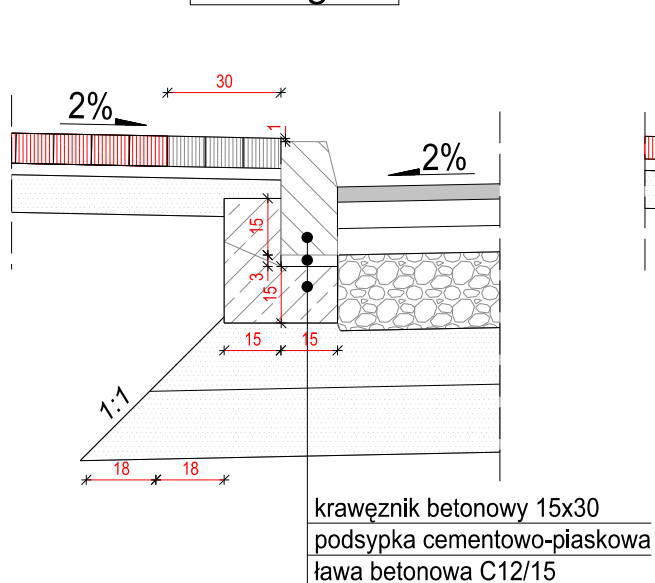
Szczegół 2
