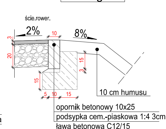
Szczegół 6
