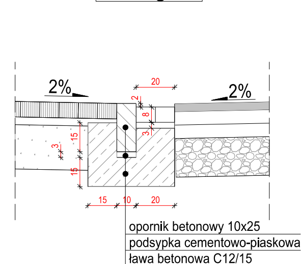
Szczegół 4
