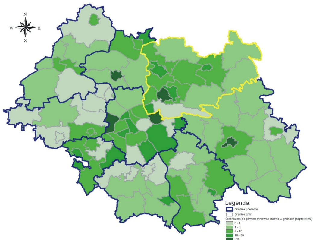
RYS. 9 EMISJA PYŁU PM 10 Z KOMUNIKACJI RAZEM Z EMISJĄ Z LICZNYCH, MAŁYCH ROZPROSZONYCH ŹRÓDEŁ EMISJI (EMISJA POWIERZCHNIOWA) UŚREDNIONA DO OBSZARU GMINY
