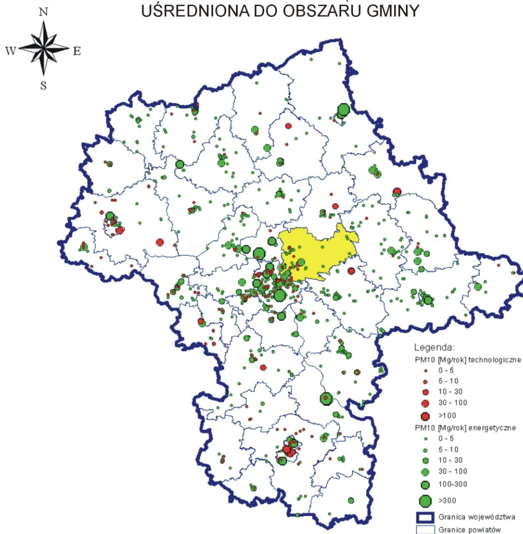
RYS. 10 LOKALIZACJA EMITORÓW PUNKTOWYCH I WIELKOŚCI EMISJI PYŁU PM 10 W WOJEWÓDZTWIE MAZOWIECKIM
