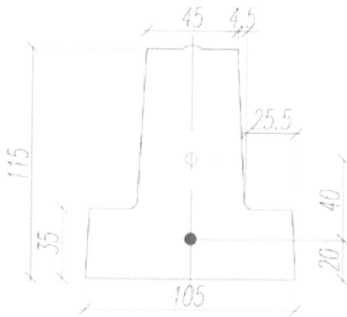
Rys. nr 2 – przekrój belki stropowej
