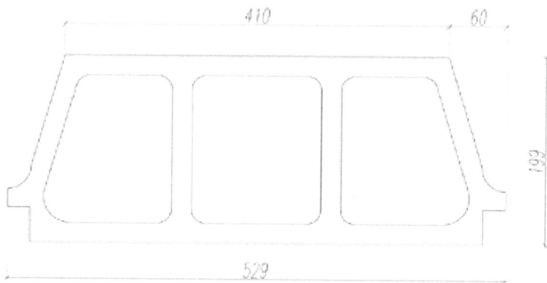
Rys. nr 3 – przekrój pustaka stropowego
